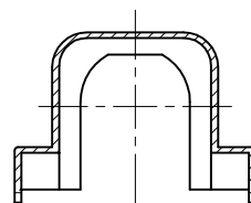
A-A SECTION
